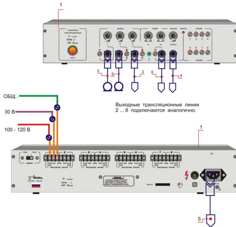
Рис. 3 Схема подключения усилителя
