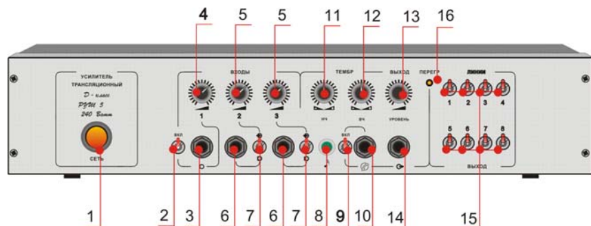
Рис. 1 Расположение органов управления на лицевой панели
