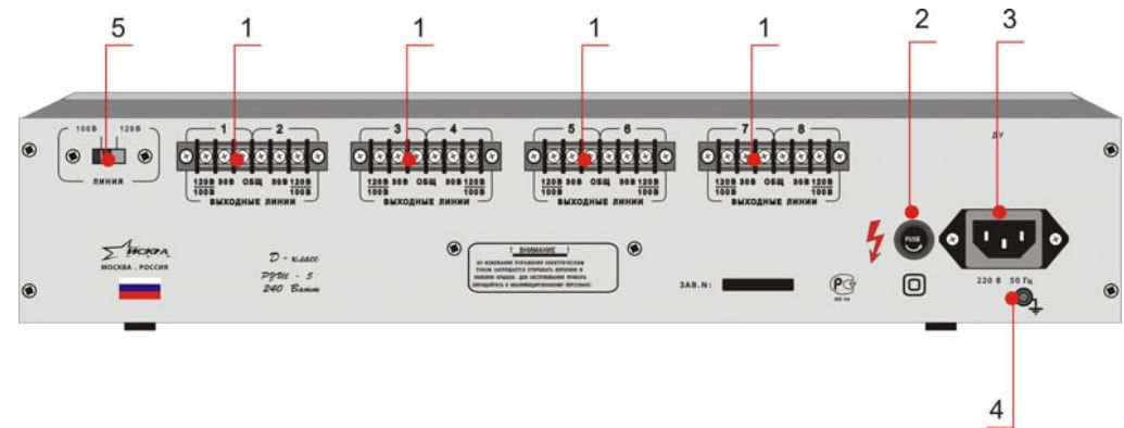
Рис. 2 Расположение органов управления на задней панели
