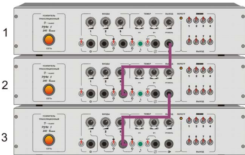
Пример каскадного включения усилителей РУШ - 5М
